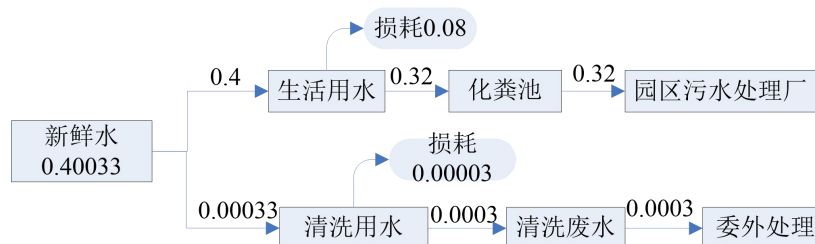
图 2-1 项目水平衡图 (单位： \text{m}^3/\text{d} )
